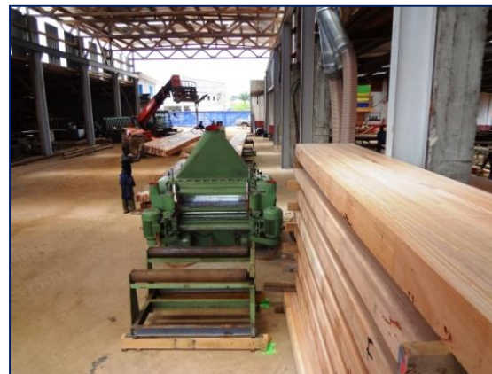
Raboteuse-4-faces jusqu'à 1.35 m de large
